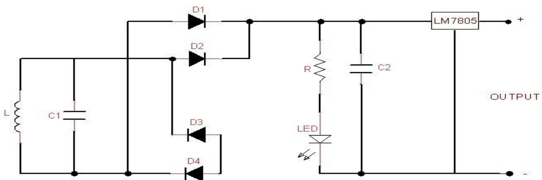
Gambar 3: Sirkuit bagian penerima
