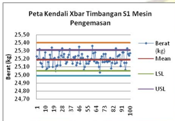
Gambar 2 Peta Kendali Xbar Timbangan S1
