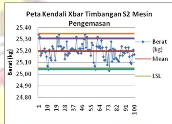
Gambar 3 Peta Kendali Xbar Timbangan S2
