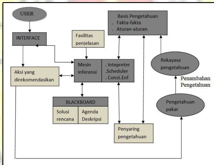
Gambar 1.1 Struktur Sistem Pakar(Kusumadewi, 2003:113-115)
