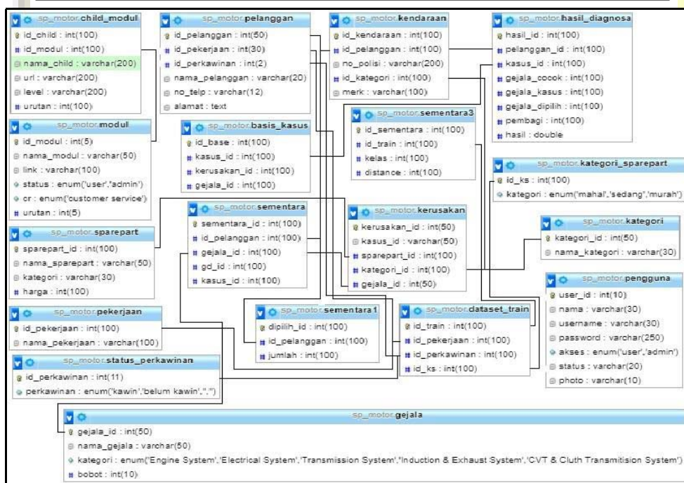
Gambar 1.8 Relasi Database
