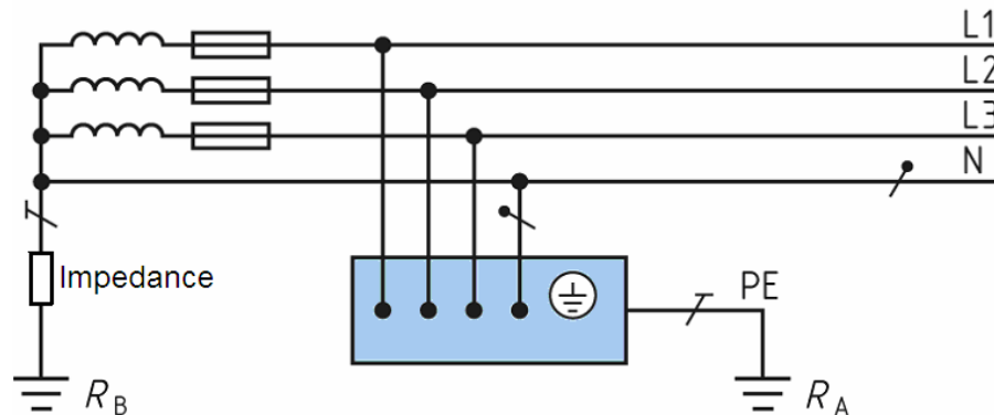
Gambar 5. Saluran Tanah Melalui Impedansi (IT)
