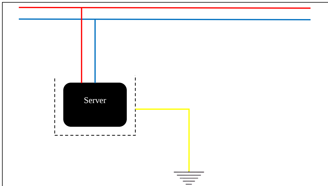
Gambar 6. Rangkaian jalur pentanahan server
