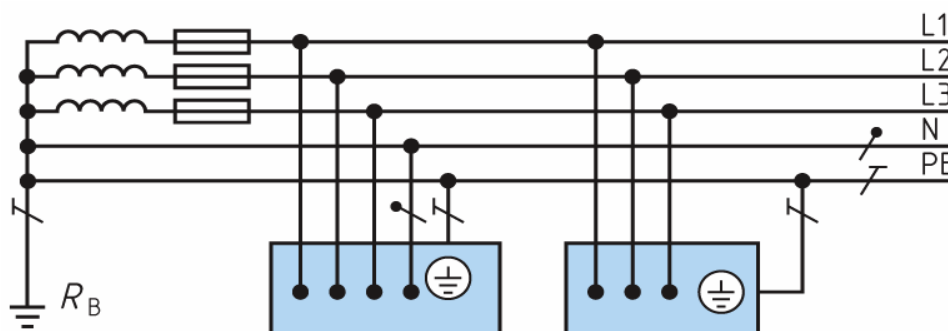
Gambar 3. Saluran Tanah dan Netral dipisah (TN-S)
