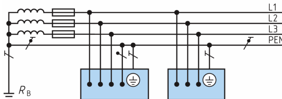
Gambar 1. Saluran Tanah dan Netral disatukan (TN-C)
