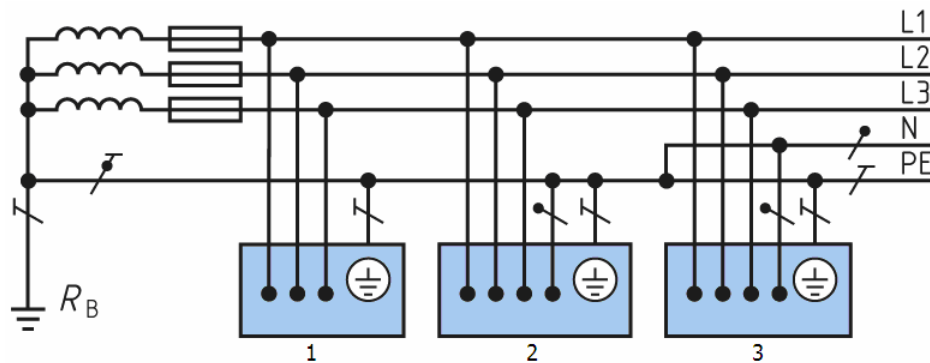
Gambar 2. Saluran Tanah dan Netral disatukan pada sebagian sistem (TN-C-S)
