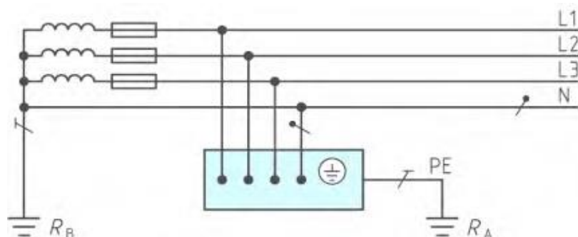
Gambar 4. Saluran Tanah Sistem dan Saluran Bagian Sistem Terpisah (TT)
