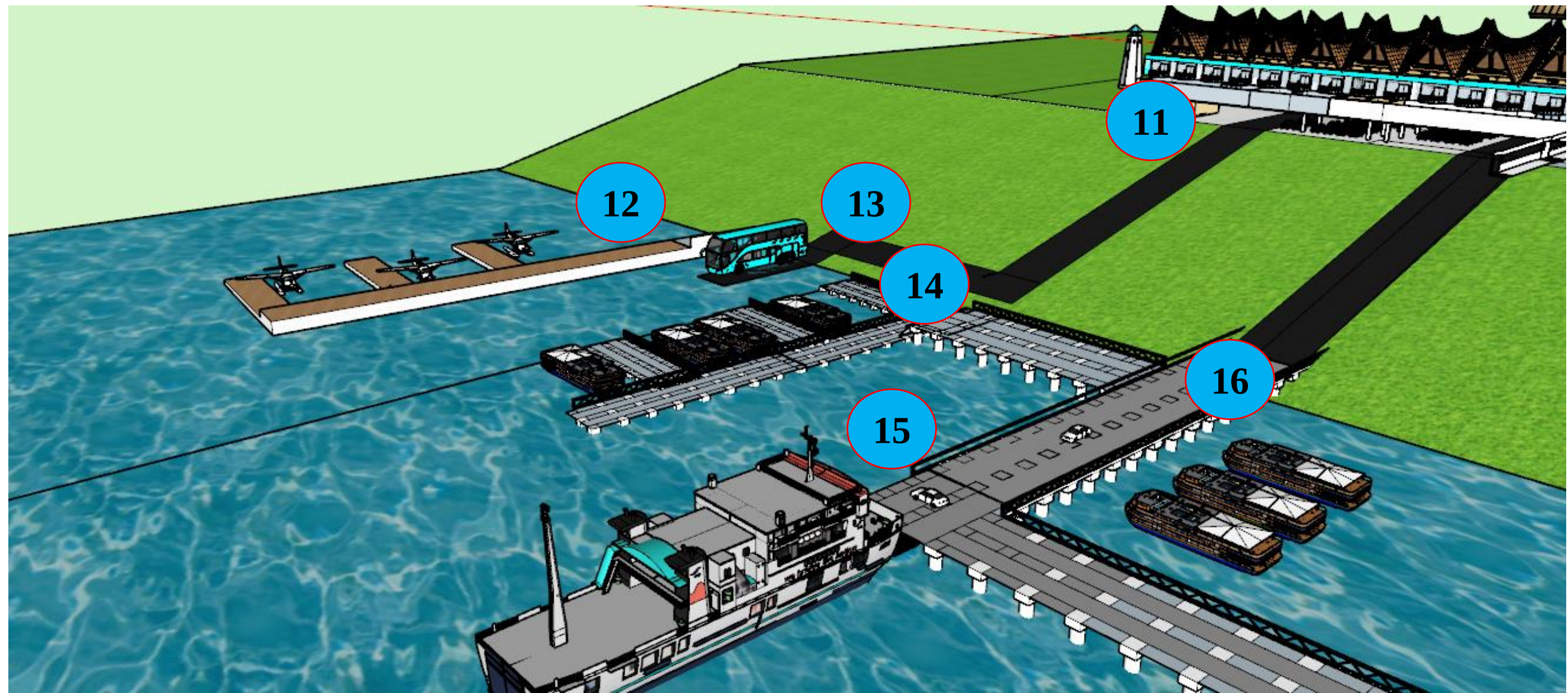
Gambar 5.32. Layout Perencanaan Pelabuhan Wisata di Perairan
