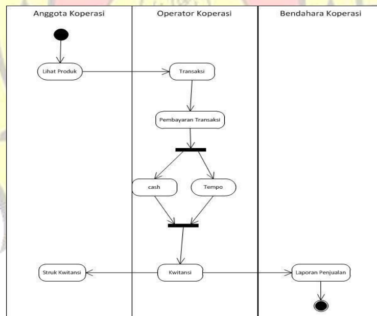
Gambar 1. Activity Diagram Prosedur sistem berjalan Sumber: uraian sistem berjalan oleh penulis (2021)
