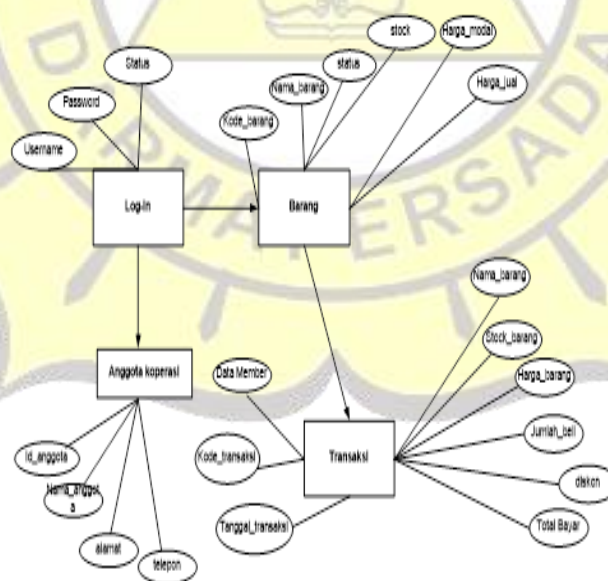
Gambar 5. Diagram ER Sumber: Perancangan Database (2021)
