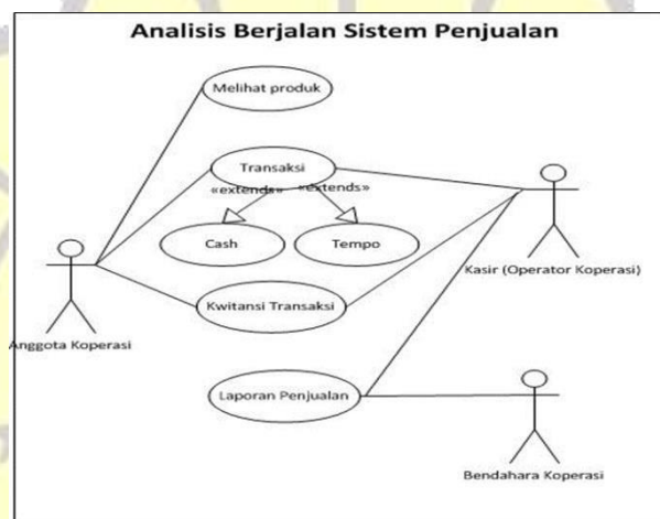
Gambar 3. Use Case Sistem Berjalan Sumber: Usecase Prosedur Sistem Usulan (2021)
