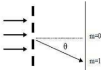
Gambar 1 Sinar datang pada kisi difraksi
