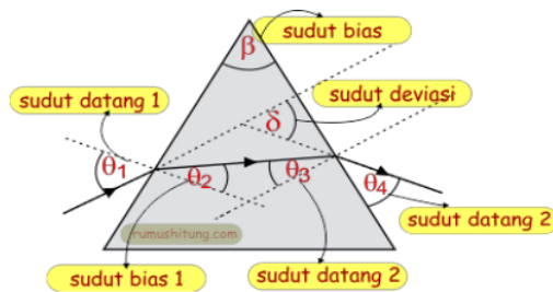
Gambar 2 Pemantulan dan Pembiasan pada Prisma
