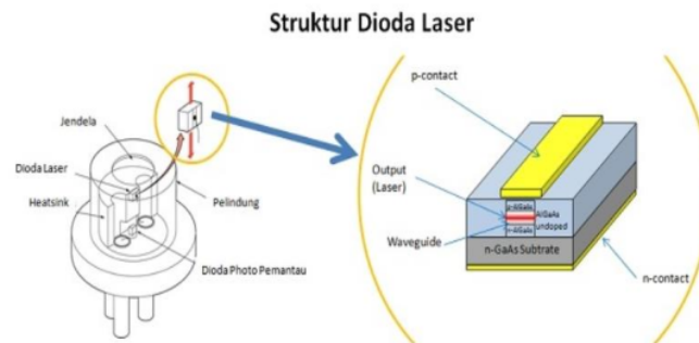
Gambar 4 Struktur diode Laser
