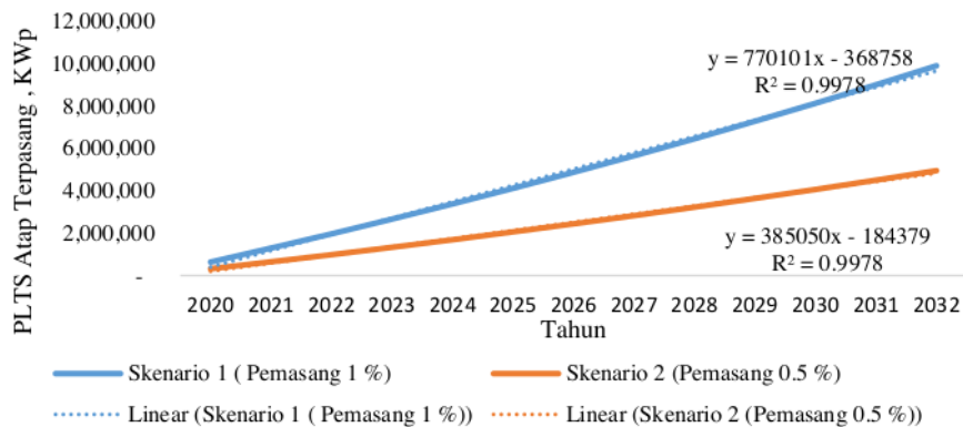
Gambar 2. Potensi Pemasangan PLTS Atap Pelanggan Rumah Tangga
