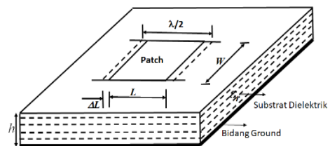
Gambar 4. Sebuah Patch Persegi.
