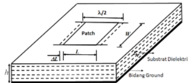
Gambar 4. Sebuah Patch Persegi.
