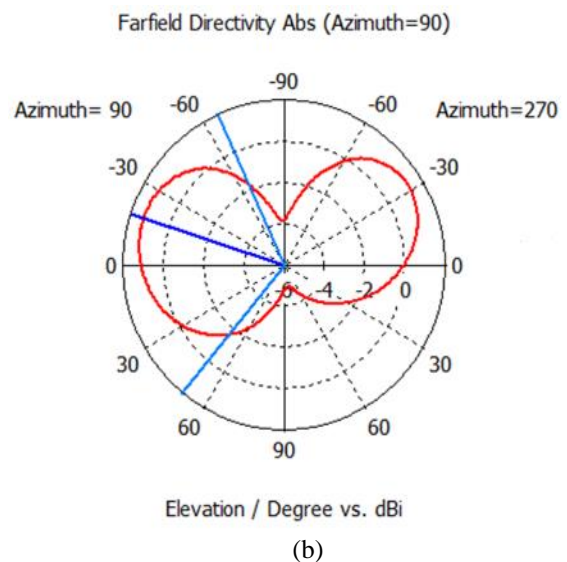
Gambar 12. Pola radiasi saat di frekuensi resonansi 3.68GHz hasil simulasi (a) Beamwidth (b) Gain
