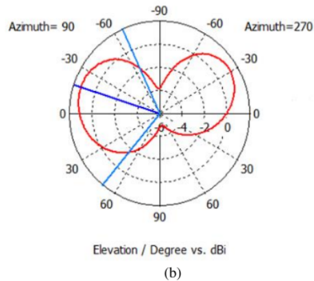
Gambar 12. Pola radiasi saat di frekuensi resonansi 3.68GHz hasil simulasi (a) Beamwidth (b) Gain
