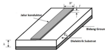
Gambar 3. Saluran Transmisi Mikrostrip.
