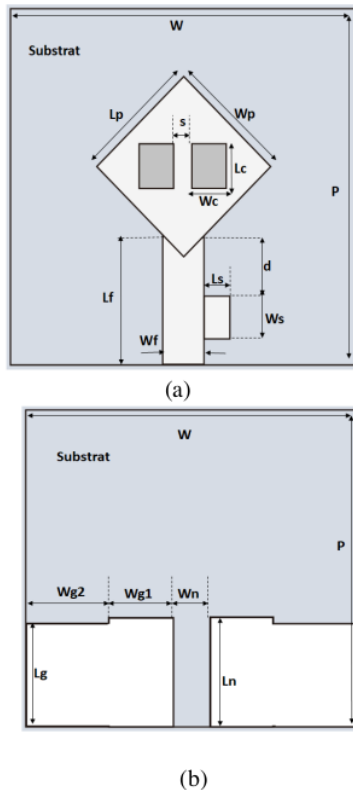
Gambar 7. Konfigurasi Rancangan Antena.
