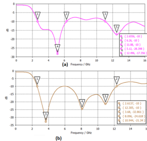
Gambar 6. Bandwidth Return loss (a) Simulasi (b) Optimasi.
