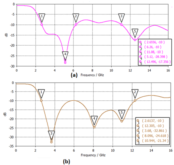
Gambar 6. Bandwidth Return loss (a) Simulasi (b) Optimasi.
