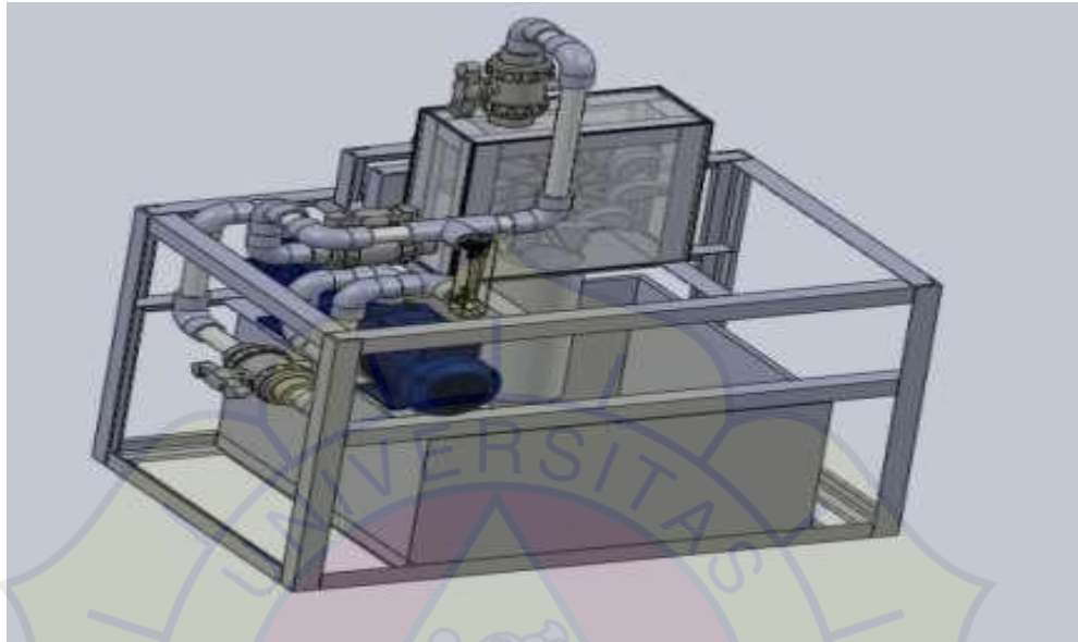
Gambar 5.1 desain rangka
