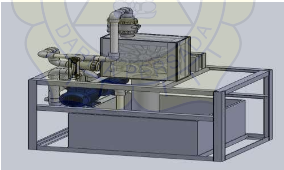
Gambar 5.2 desain rangka
