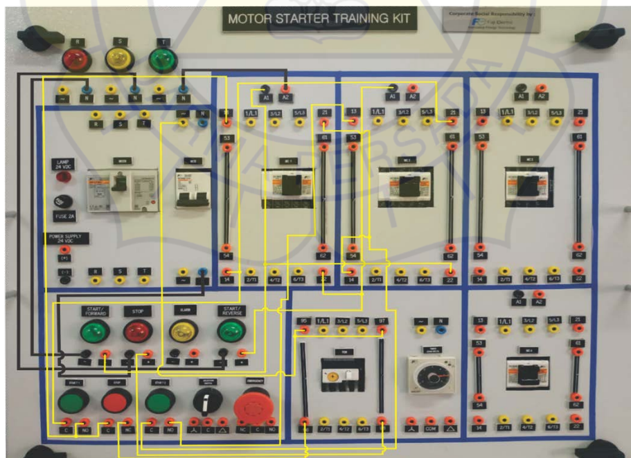
Jalur Skema Rangkaian Kontrol
