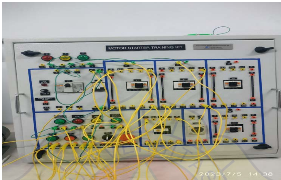
Rangkaian Kontrol
