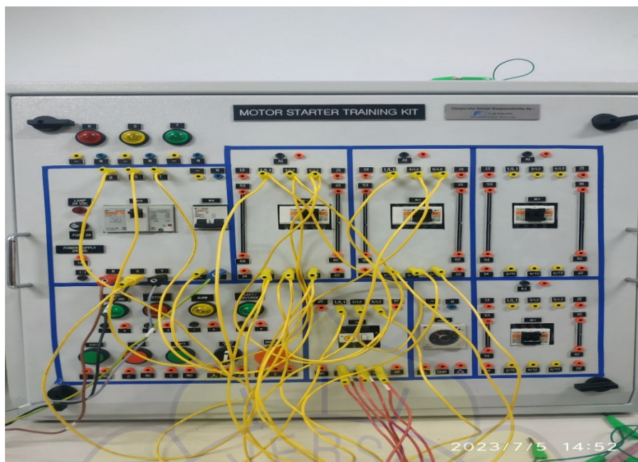
Rangkaian Daya
