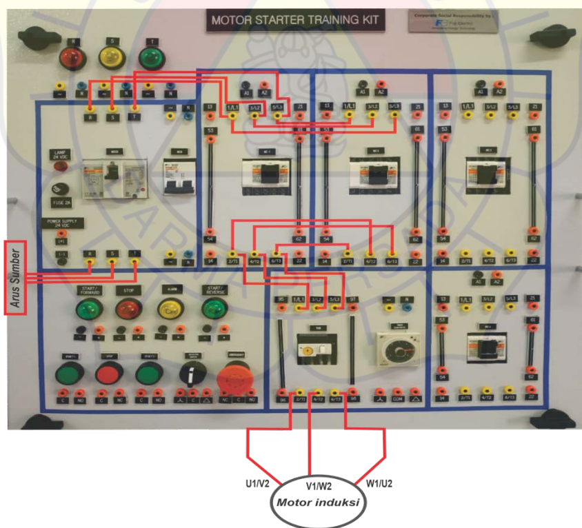
Jalur Skema Rangkaian Daya
