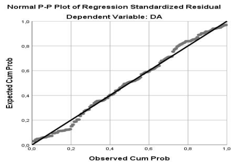
Grafik Normalitas
